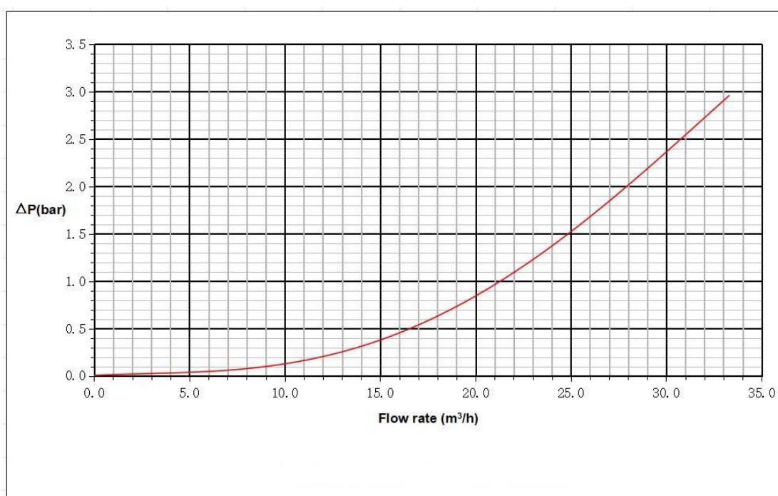
Рисунок 1 – Кривая потери давления – Режим фильтрации
