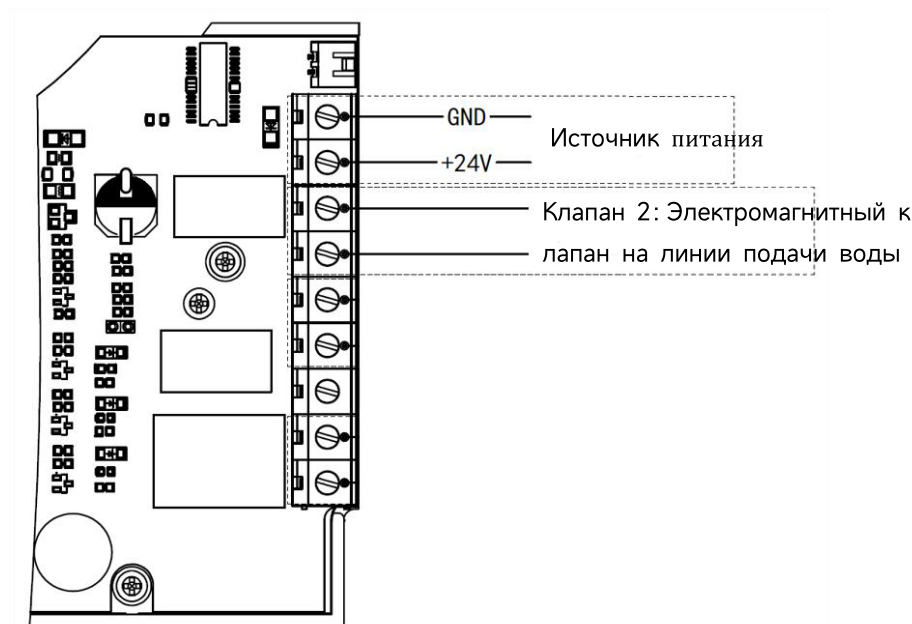
Рисунок 9 - Схема подключения электромагнитного клапана (клапан 2)
