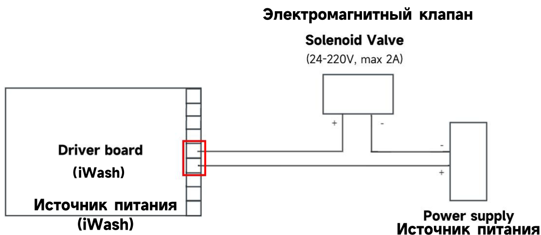
Рисунок 8 - Схема подключения электромагнитного клапана (клапан 1)
