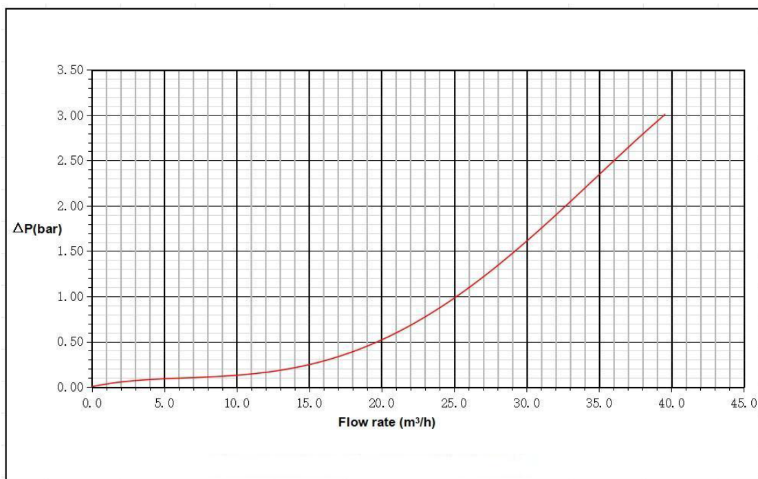
Рисунок 2 – Кривая потери давления – Режим обратной промыв
