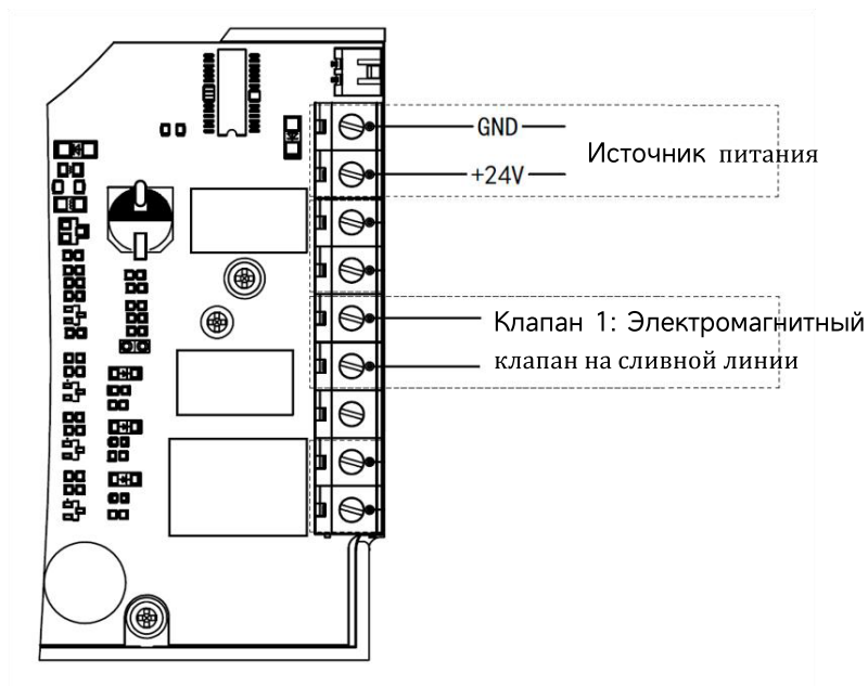
Рисунок 7 - Клеммная колодка электромагнитного клапана — Клапан 1
