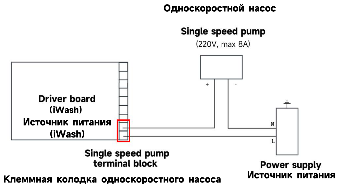
Рисунок 11 - Схема подключения односкоростного насоса (ток \leq 8A )
