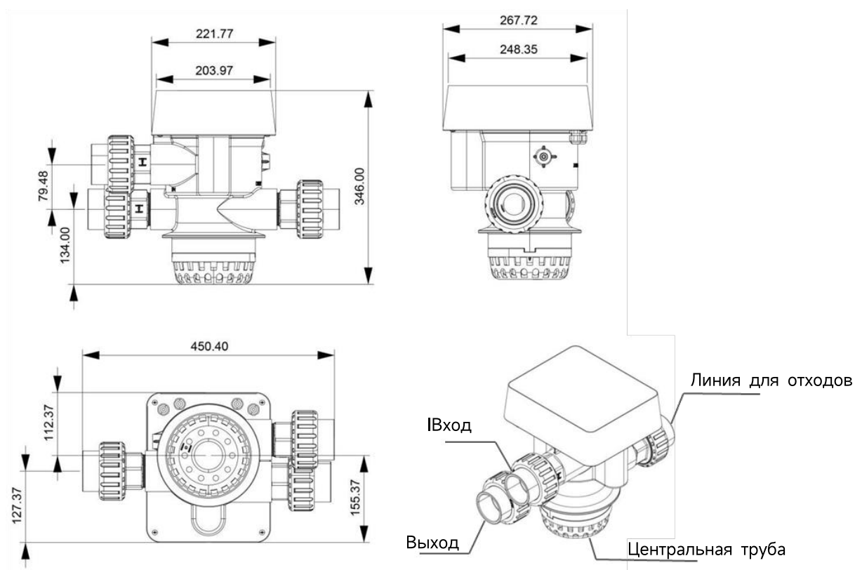
Рисунок 3 - Размеры многопортового клапана
