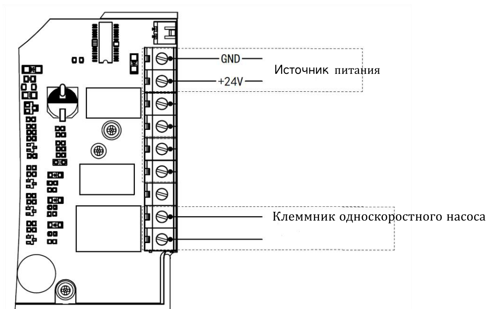
Рисунок 10 - Клеммная колодка односкоростного насоса
