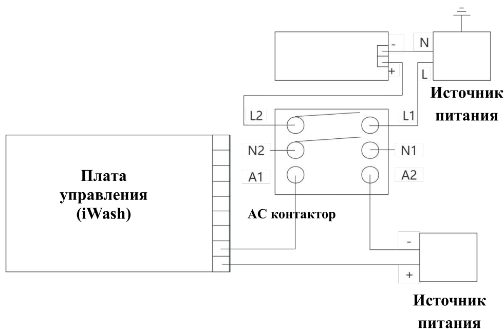
Рисунок 12 - Схема подключения односкоростного насоса (ток \leq 8A )
