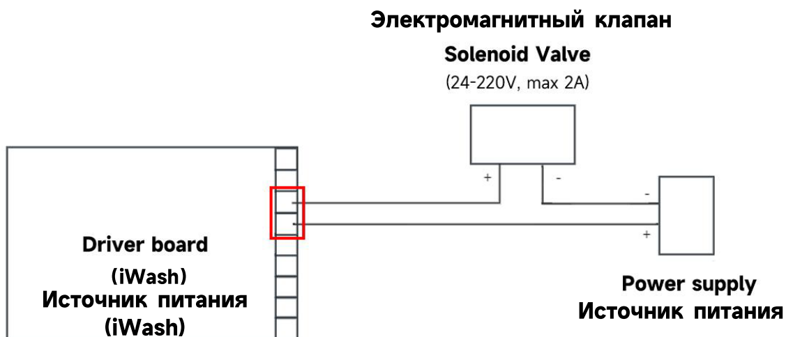
Рисунок 9 - Схема подключения электромагнитного клапана (клапан 2)
