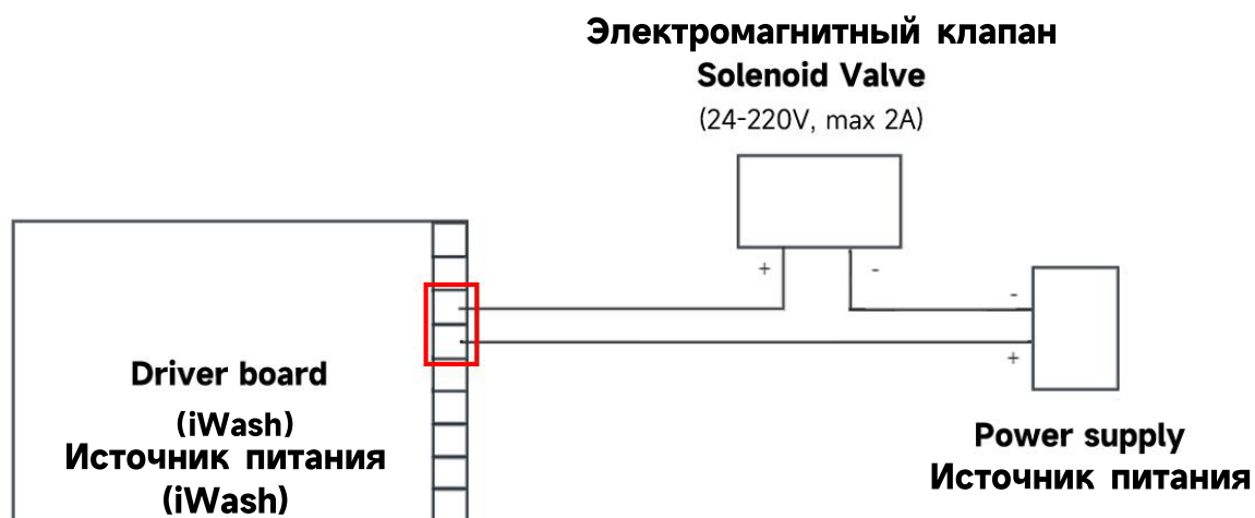
Рисунок 9 - Схема подключения электромагнитного клапана (клапан 2)
