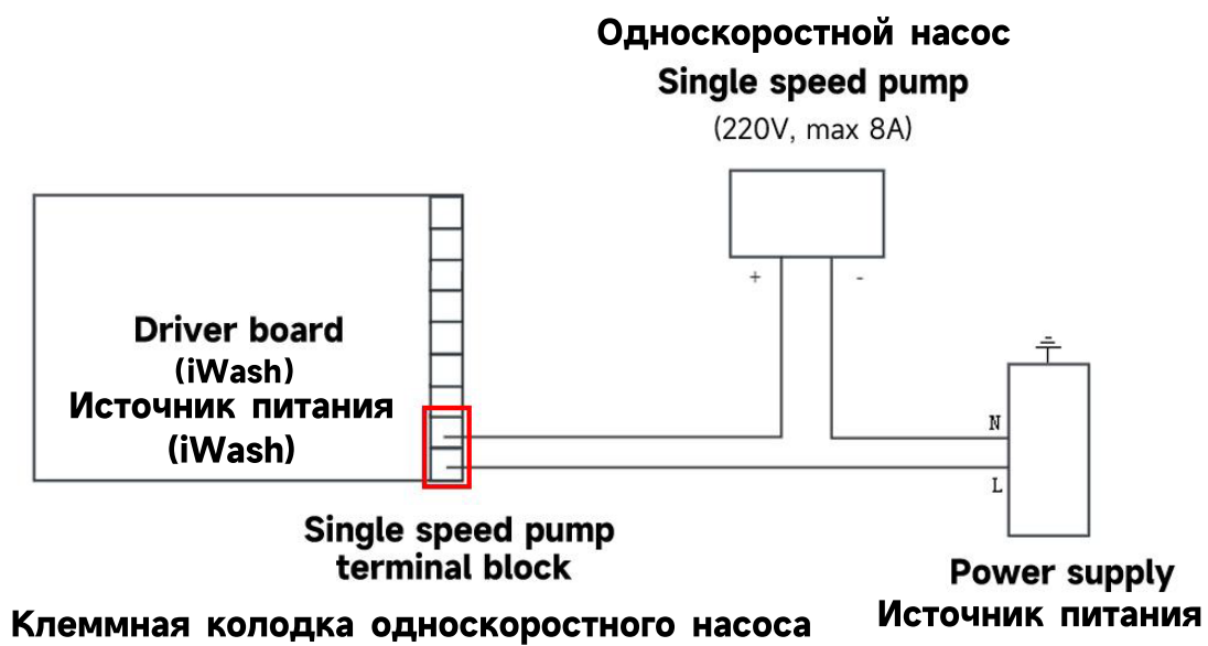
Рисунок 12 - Схема подключения односкоростного насоса (ток \leq 8A )
