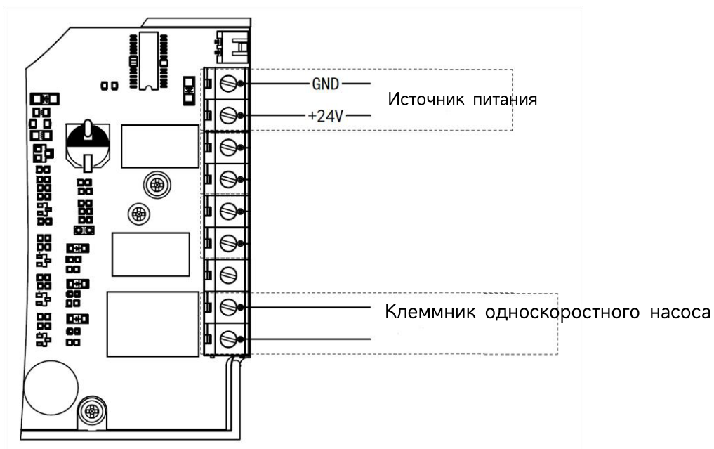
Рисунок 11 - Клеммная колодка односкоростного на
