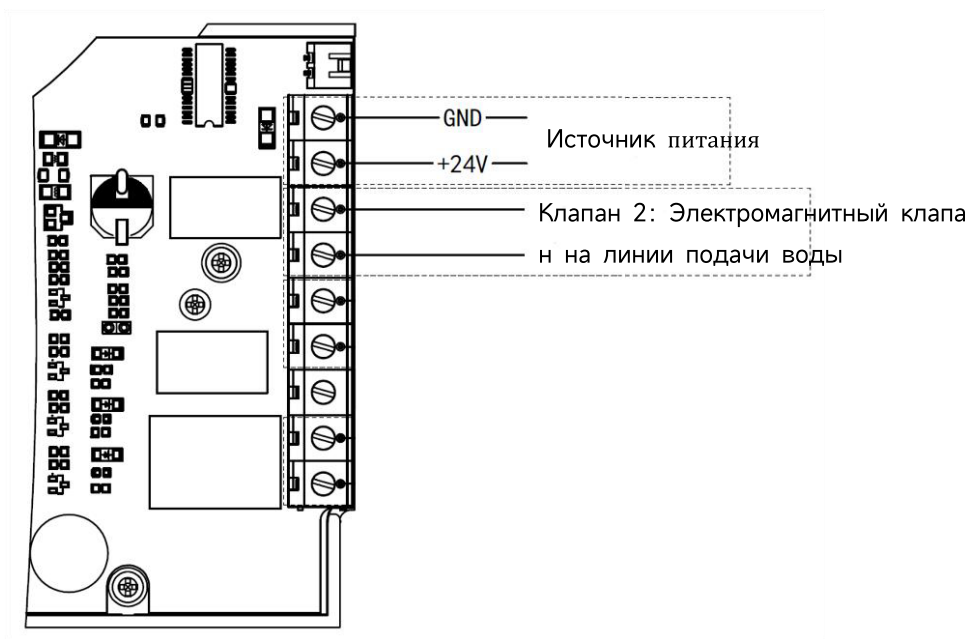
Рисунок 9 - Схема подключения электромагнитного клапана (клапан 2)
