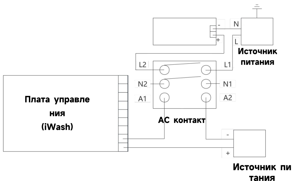
Рисунок 13 - Схема подключения односкоростного насоса (ток \leq 8A )
