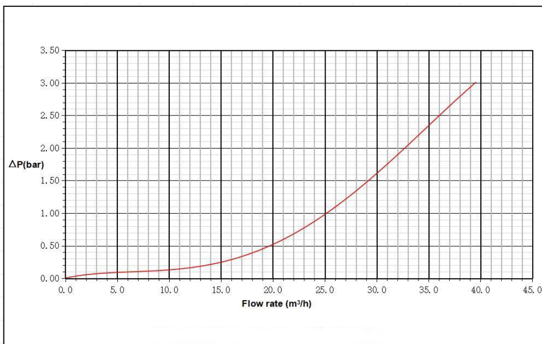
Рисунок 2 – Кривая потери давления – Режим обратной про
