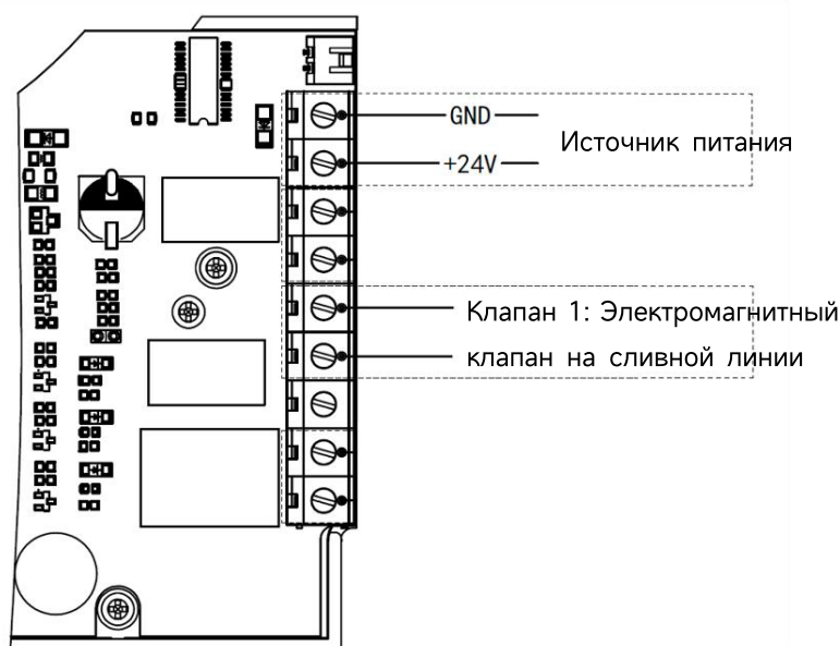
Рисунок 7 - Клеммная колодка электромагнитного клапана — Клапан 1
