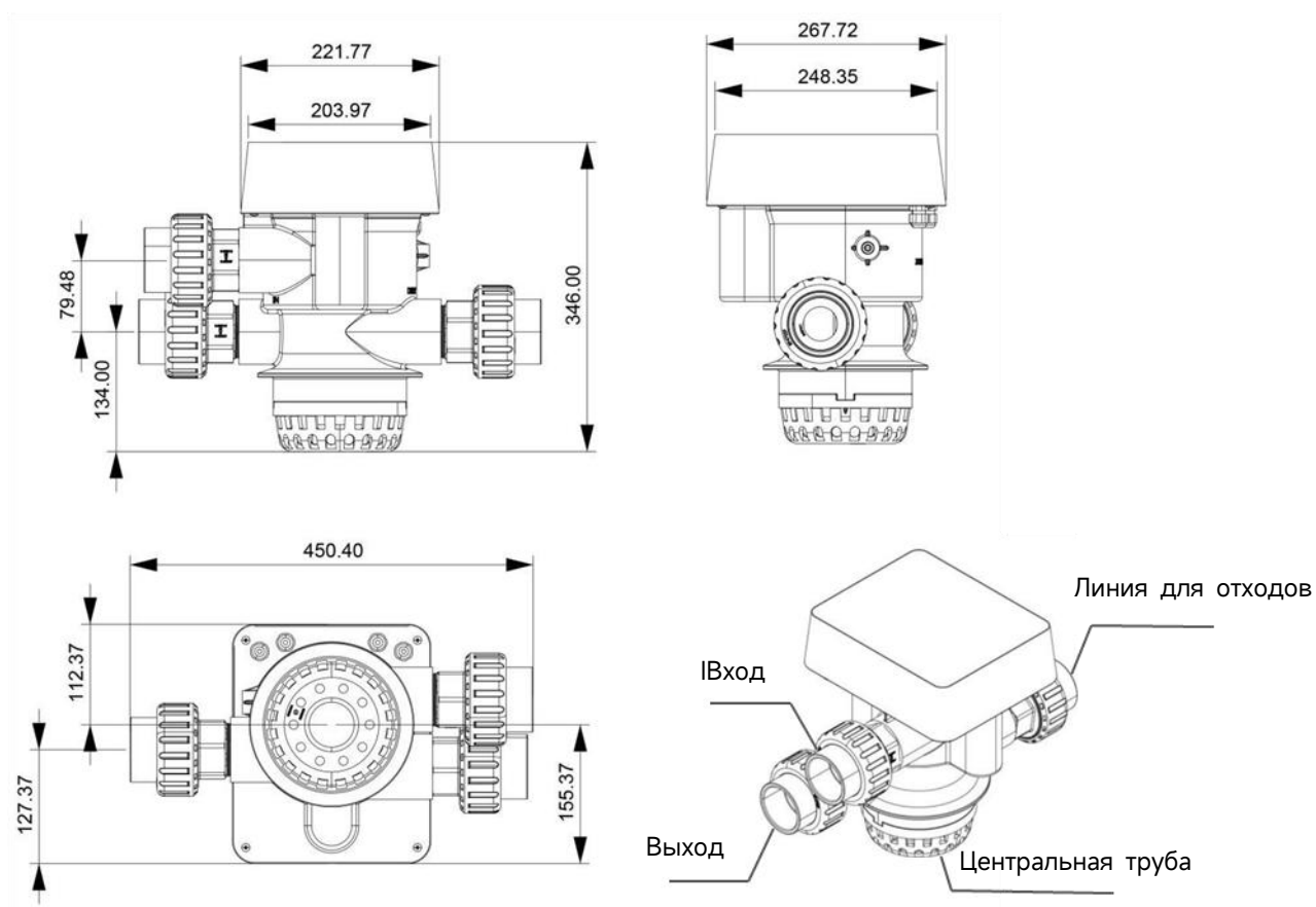
Рисунок 3 - Размеры многопортового клапана
