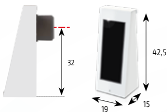
ROLLEASY 2 ЭЛЕКТРОПРИВОД / СОЛНЕЧНАЯ БАТАРЕЯ (до 5 м шириной)
