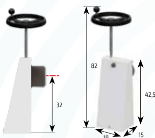
ROLLEASY 2 РУЧНОЙ ПРИВОД
