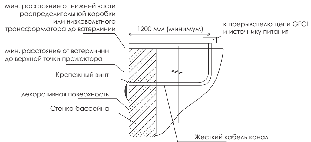
Схема монтажа
